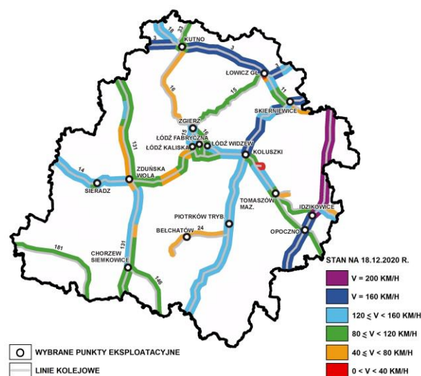
Rys. 50. Maksymalne prędkości na liniach kolejowych, stan na 18.12.2020 r.
